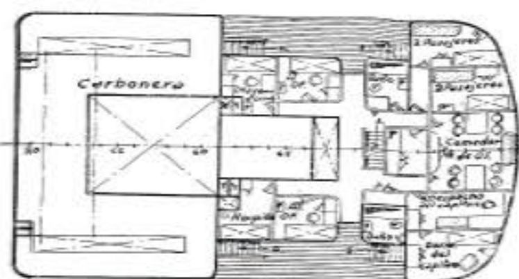
CUBIERTA DE CIUDADELA
